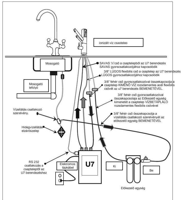
Telepítési ábra
